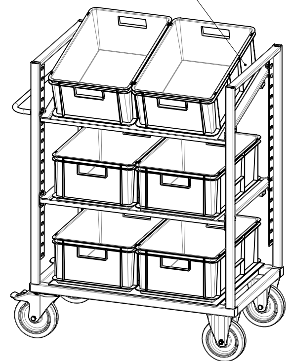
KLT-Kiste 600x400x220
