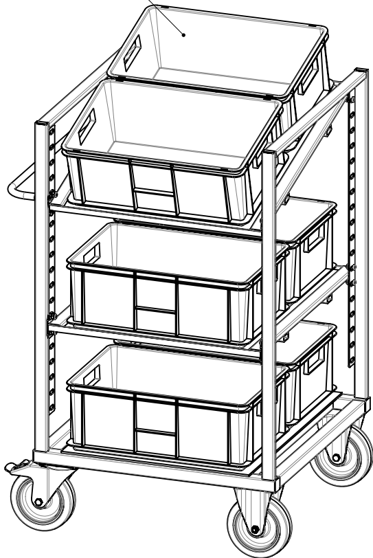
KLT-Kiste 600x400x220
